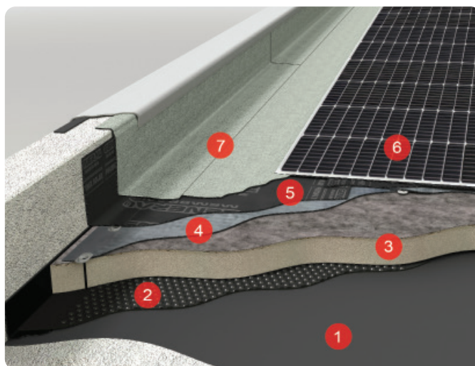
Fig. 4 Stratigrafia esemplificativa: Sistema General Solar PV su manto bituminoso
