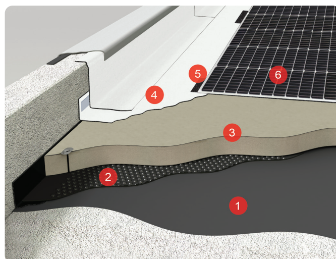
Fig. 5 Stratigrafia esemplificativa: Sistema General Solar PV SH su manto sintetico
